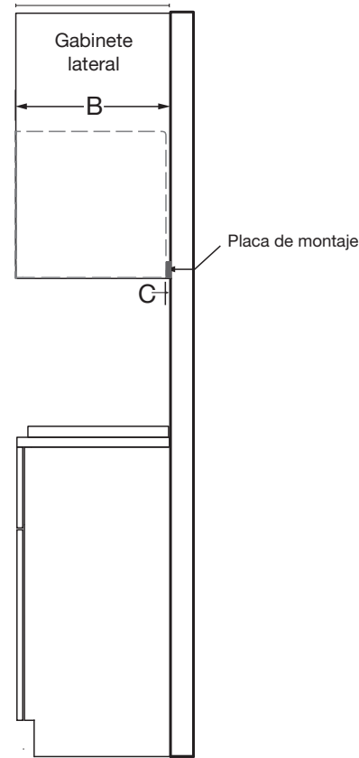
VISTA LATERAL
