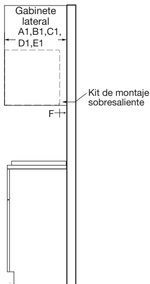
VISTA LATERAL
